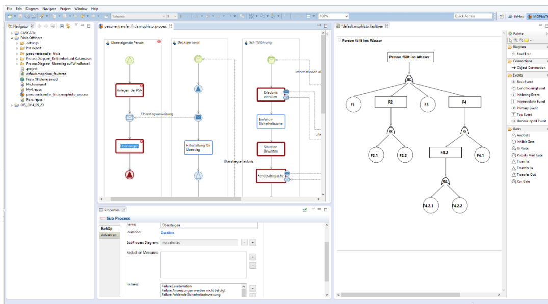
Abbildung 46: MOPhisTo - Fehlerbaumeditor
