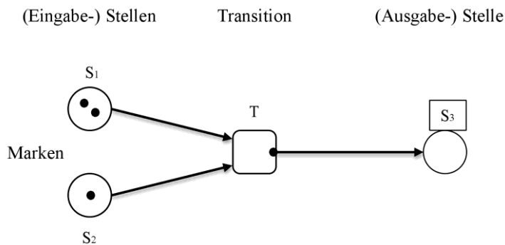
Abbildung 12: Beispiel eines Petri-Netzes
