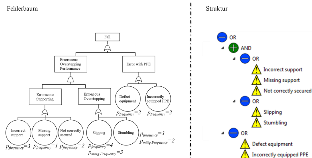
Abbildung 53: Auszug aus der Gesamtdokumentation und dem zugehörigen Fehlerbaum zu der Gefährdung "Sturz" [Pi15]
