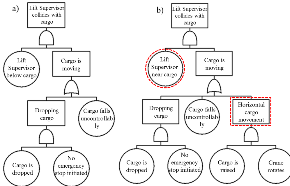
Abbildung 60: Fehlerbäume des Verladeszenarios. a) vor b) nach der simulationsbasierten Analyse
