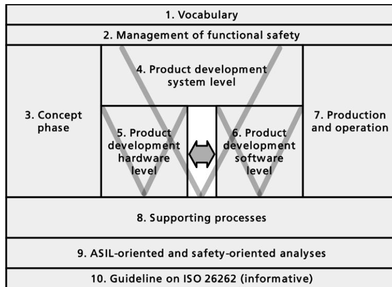
Abbildung 4: Vereinfachtes Lebenszyklusmodell der ISO 26262 [In08]
