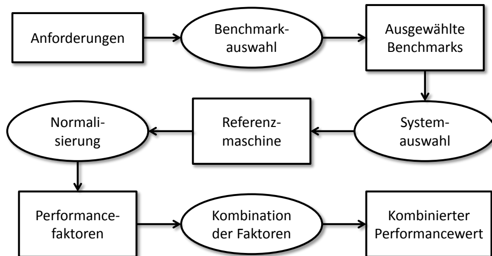
Abbildung 4.7: Prinzipieller Ablauf der Performancemodellierung von Server- und Stagesystemen
