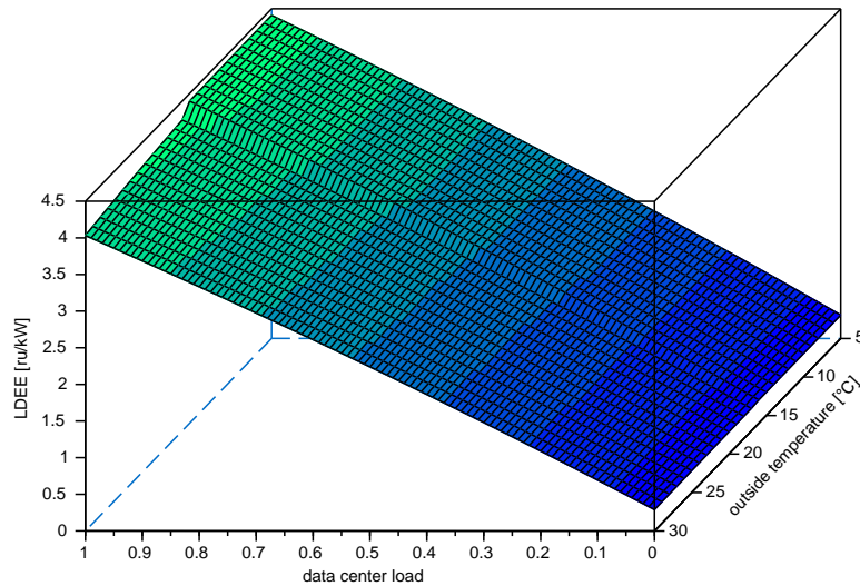
Abbildung 3.1: Verlauf der LDEE eines nicht optimierten Betriebs
